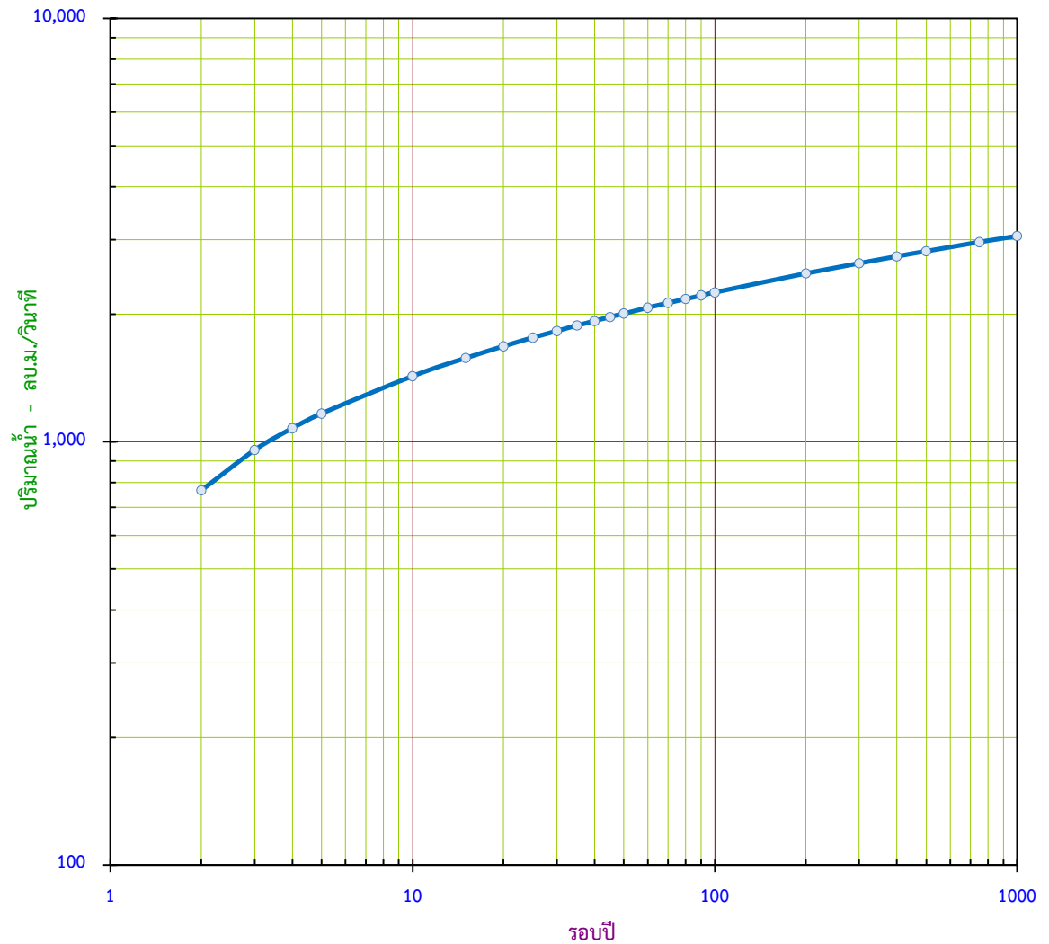
กราฟแสดง ปริมาณน้ำสูงสุดรายปี ขนาดรอบปีต่างๆ สถานี N.5A ในเมือง อ.เมือง จ.พิษณุโลก
